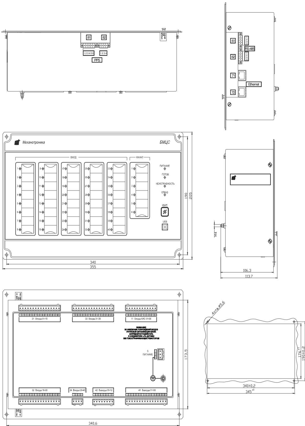
Рисунок 8 - Габаритные и установочные размеры блока
