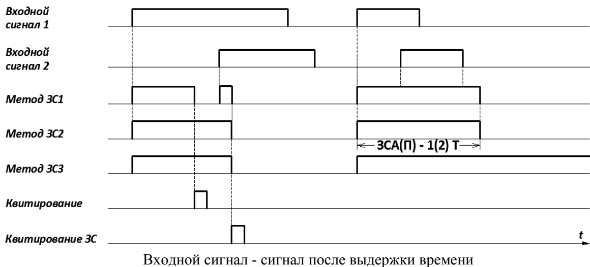
Рисунок 6 - Временные диаграммы звуковой сигнализации
