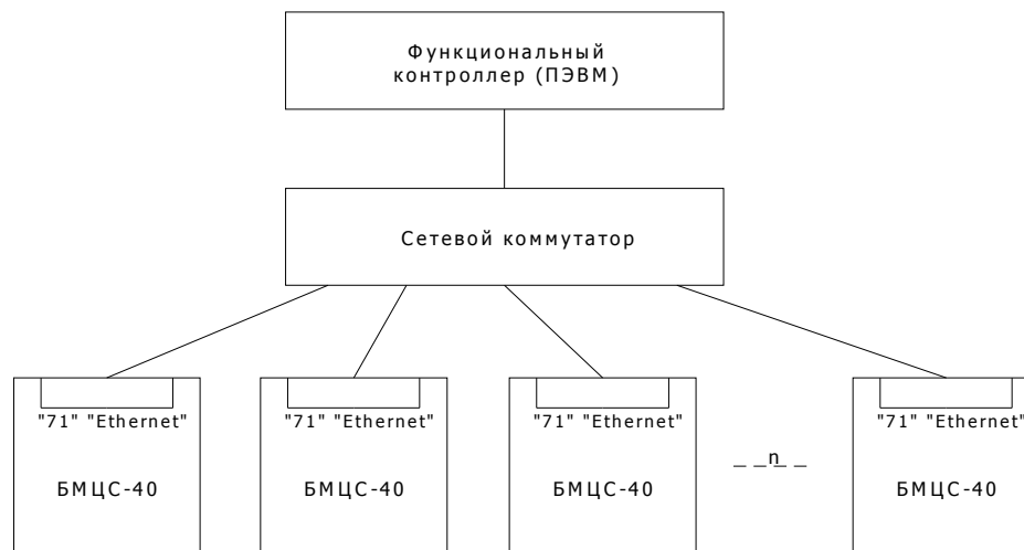
Рисунок Б.2 - Организация топологии сети (Ethernet)
