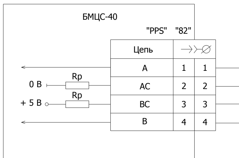
Рисунок Б.5 - Схема электрическая подключения соединителя "82" "PPS"
