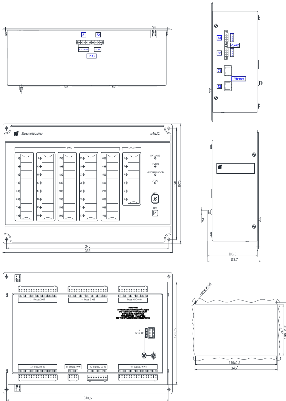
Рисунок 8 - Габаритные и установочные размеры блока
