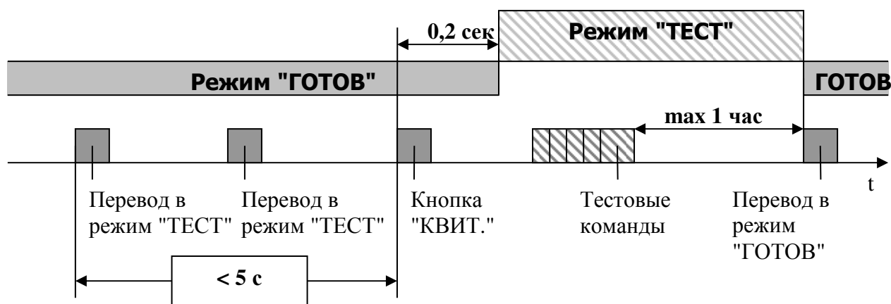
Рисунок 7 - Перевод БМЦС-40 в режим "ТЕСТ" и в режим "ГОТОВ"
