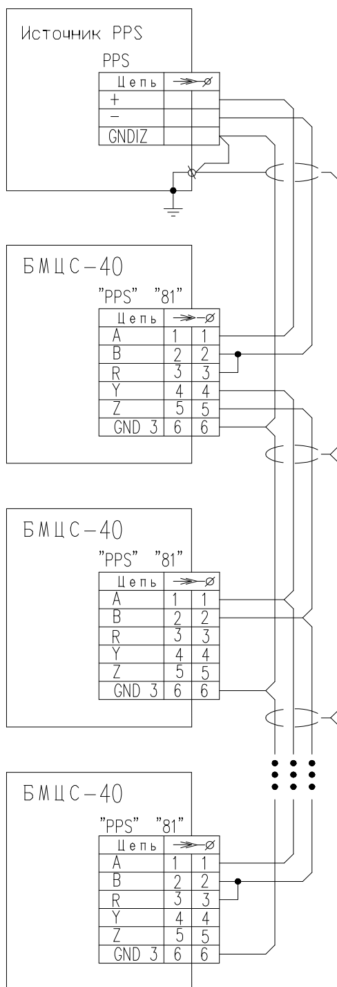
Рисунок Б.3 - Схема электрическая подключения цепей "PPS" (вариант 1)
