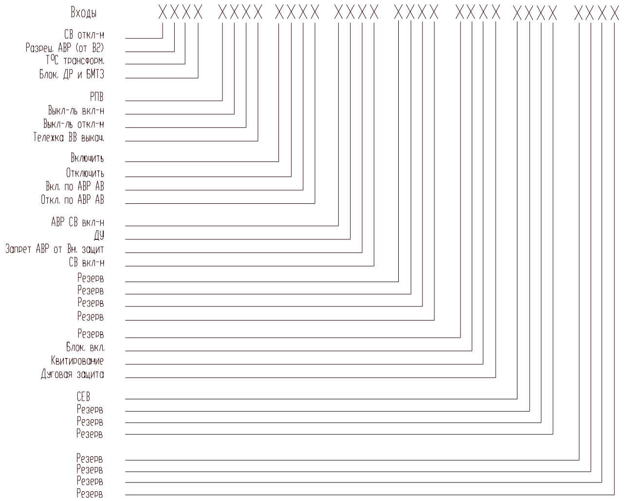
Рисунок Г.1 - Соответствие дискретных входов позициям дисплея
