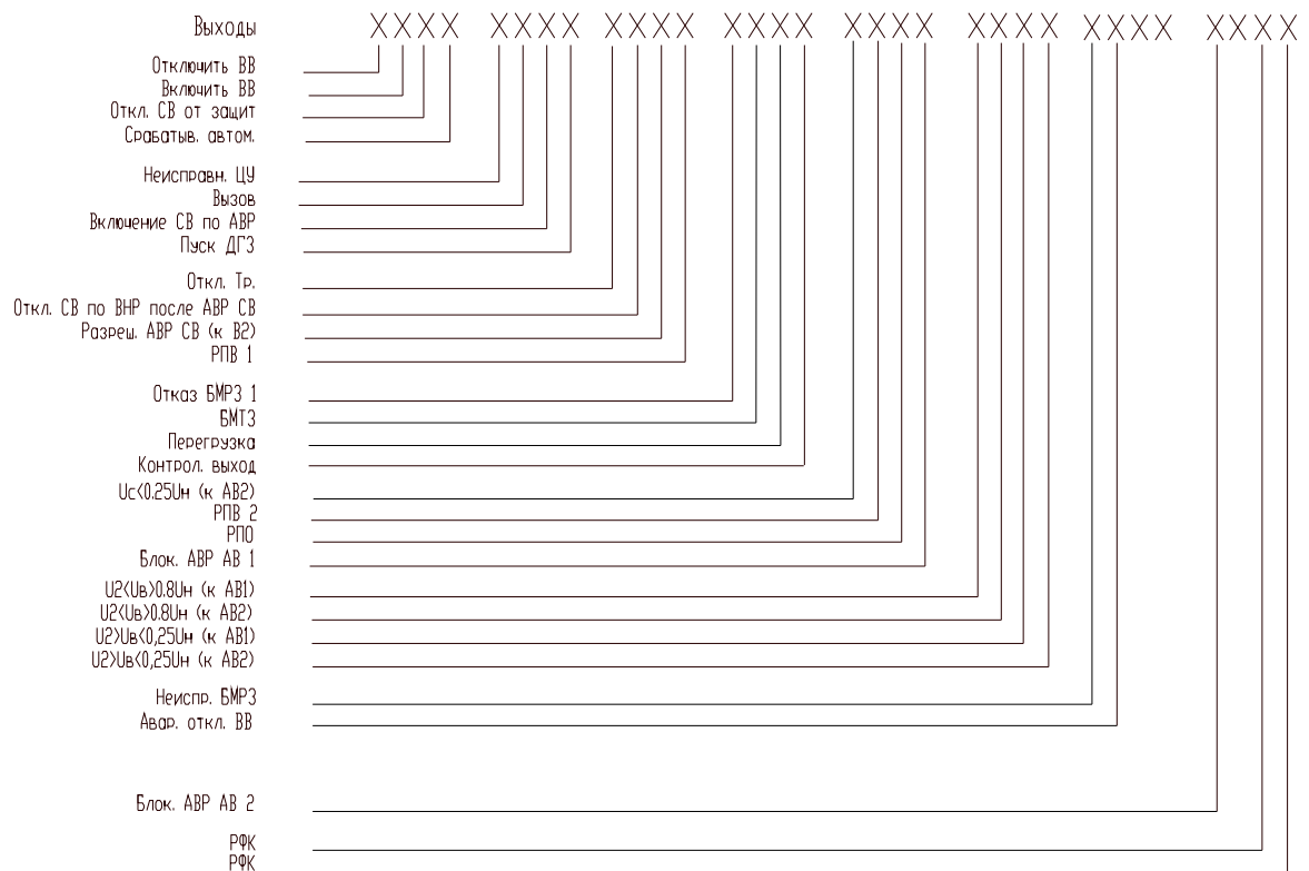
Рисунок Г.2 - Соответствие дискретных выходов позициям дисплея
