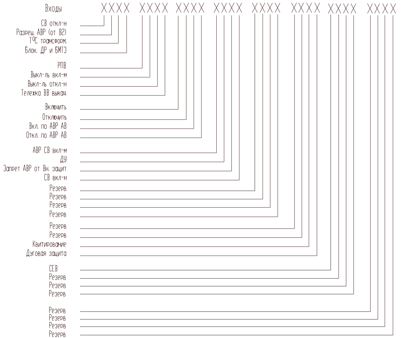
Рисунок Г.1 - Соответствие дискретных входов позициям дисплея
