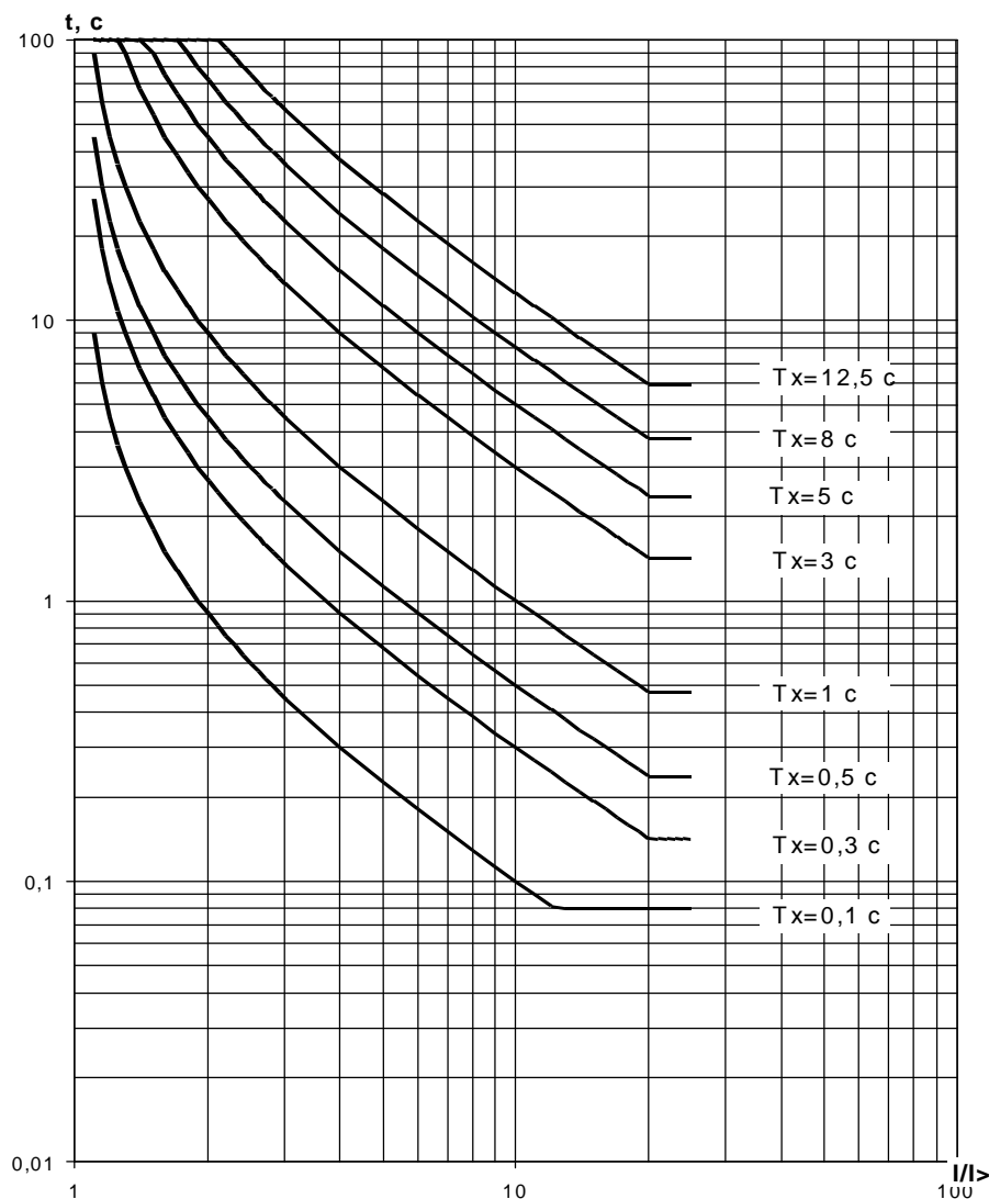
Рисунок Е.1 - Обратнозависимая времятоковая характеристика
