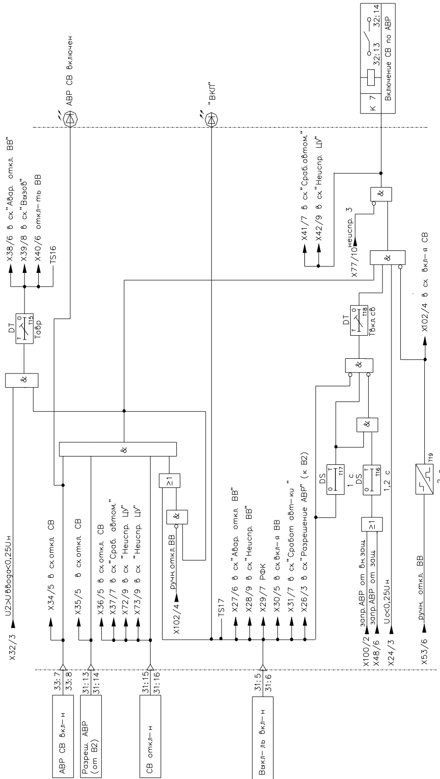
Рисунок Б.4 – Функциональная схема алгоритма "Включение CB по АВР"
