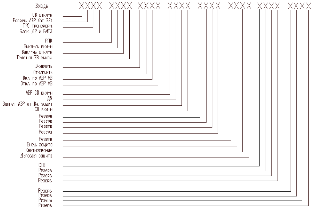
Рисунок Г.1 - Соответствие дискретных входов позициям дисплея
