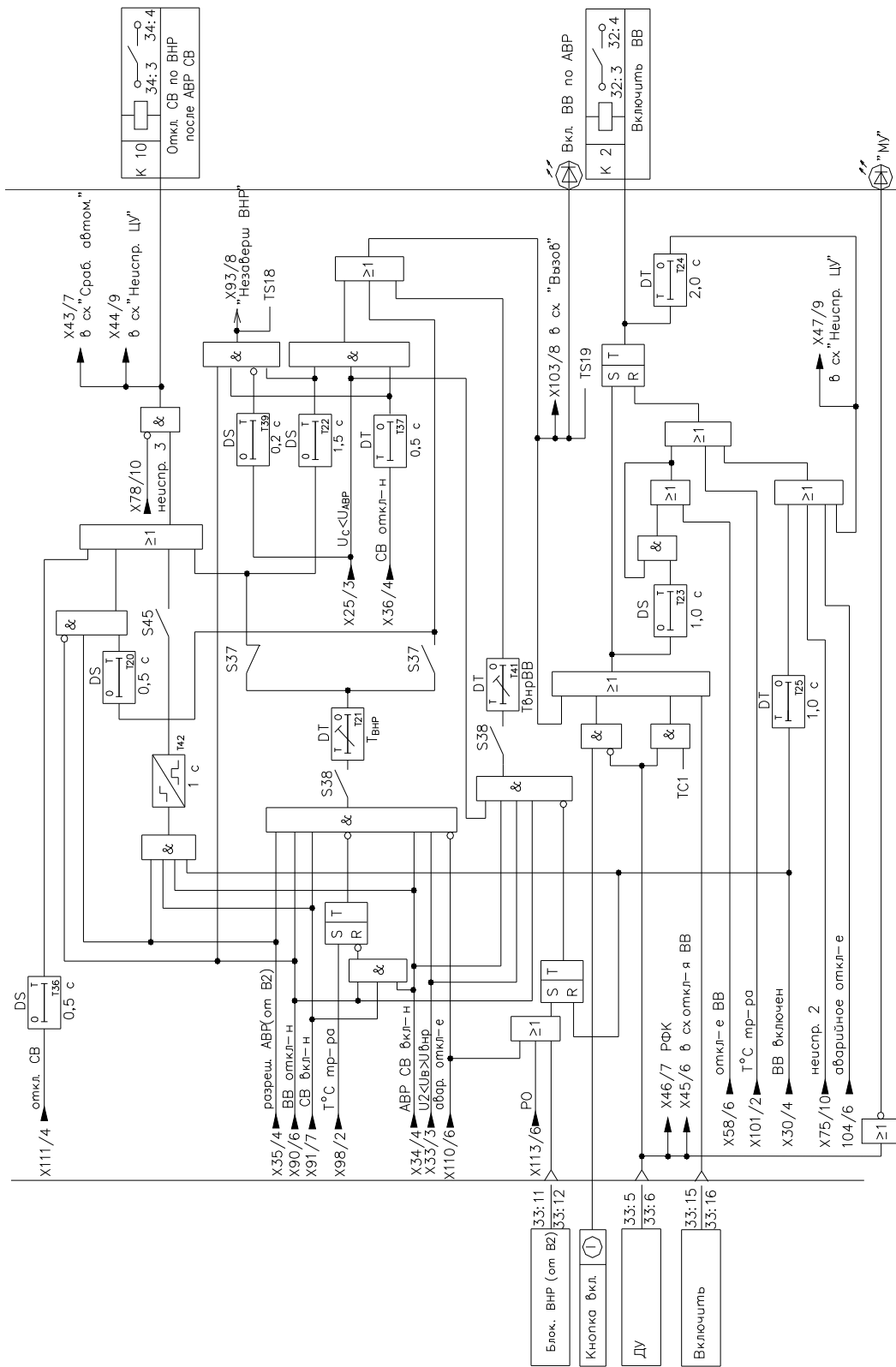
Рисунок Б.5 – Функциональная схема алгоритма отключения СВ при возврате АВР СВ и схема алгоритма "Управление выключателем – включение"
