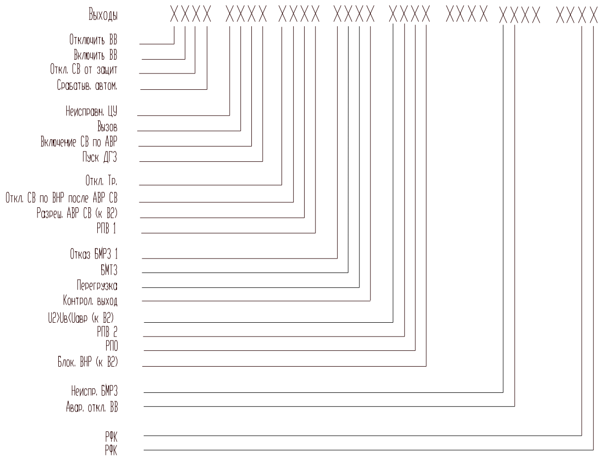
Рисунок Г.2 - Соответствие дискретных выходов позициям дисплея
