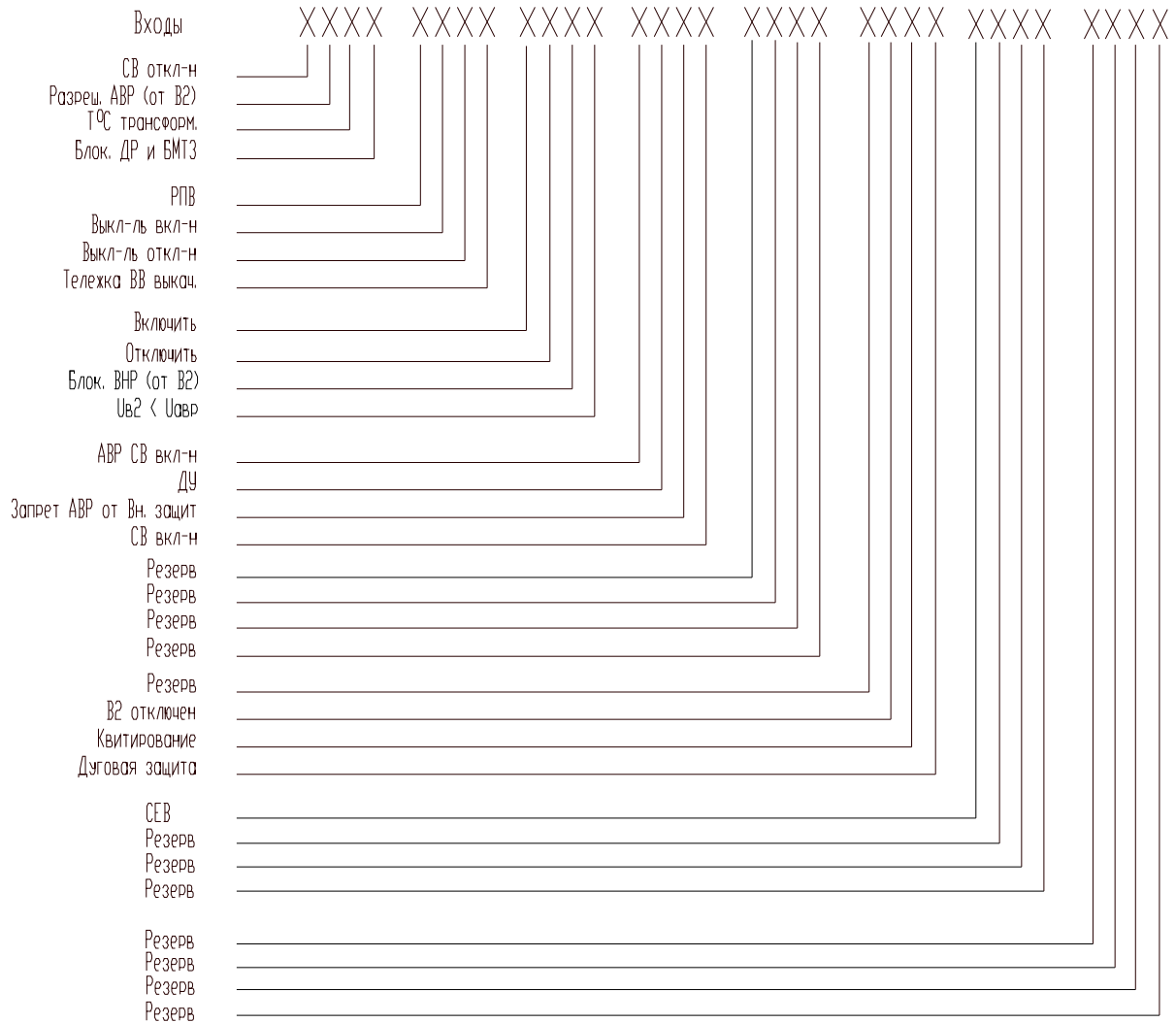
Рисунок Г.1 - Соответствие дискретных входов позициям дисплея
