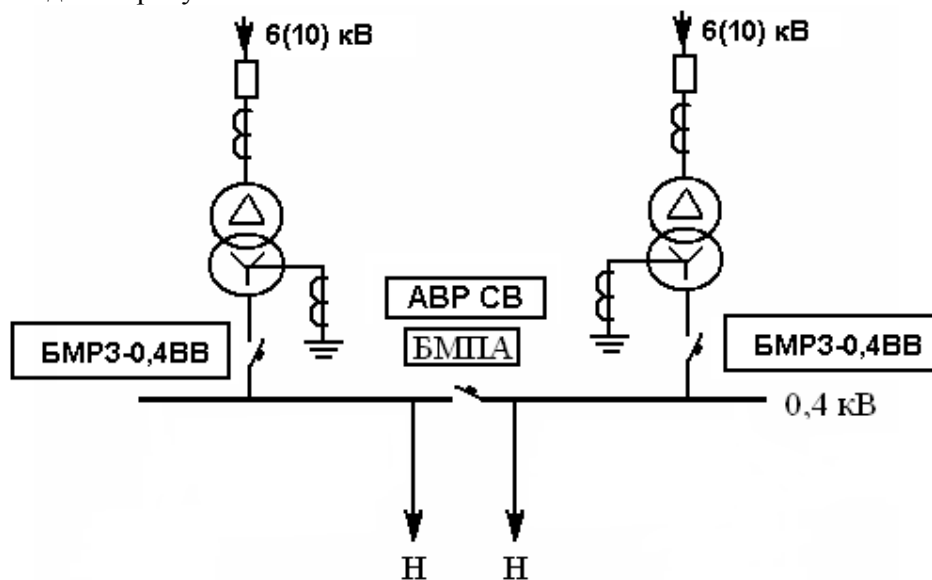
Рисунок Ж.1 - Пример структурной схемы АВР
