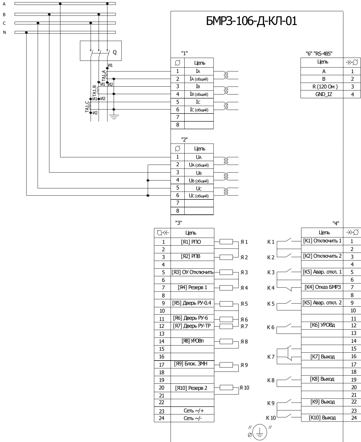
Рисунок А.1 - Схема электрическая подключения
