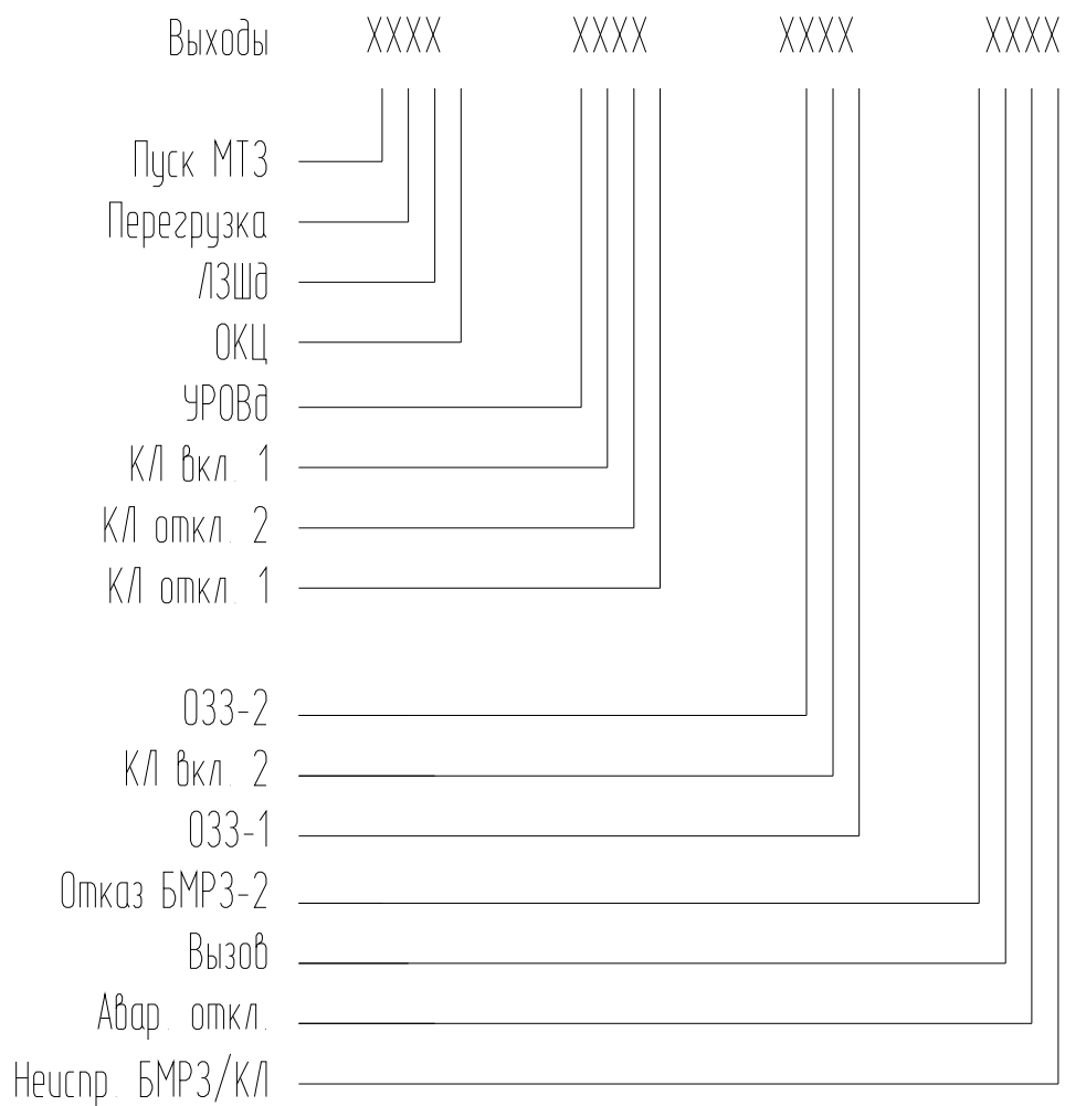
Рисунок Г.2 - Соответствие дискретных выходов позициям дисплея
