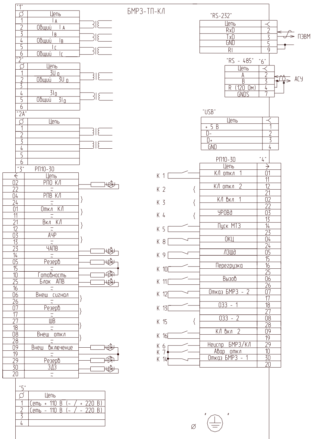
Рисунок А 1 - Схема электрическая подключения
