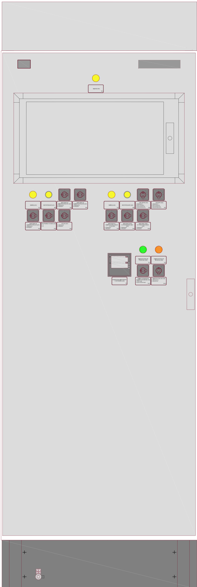
Шкаф - вид спереди
