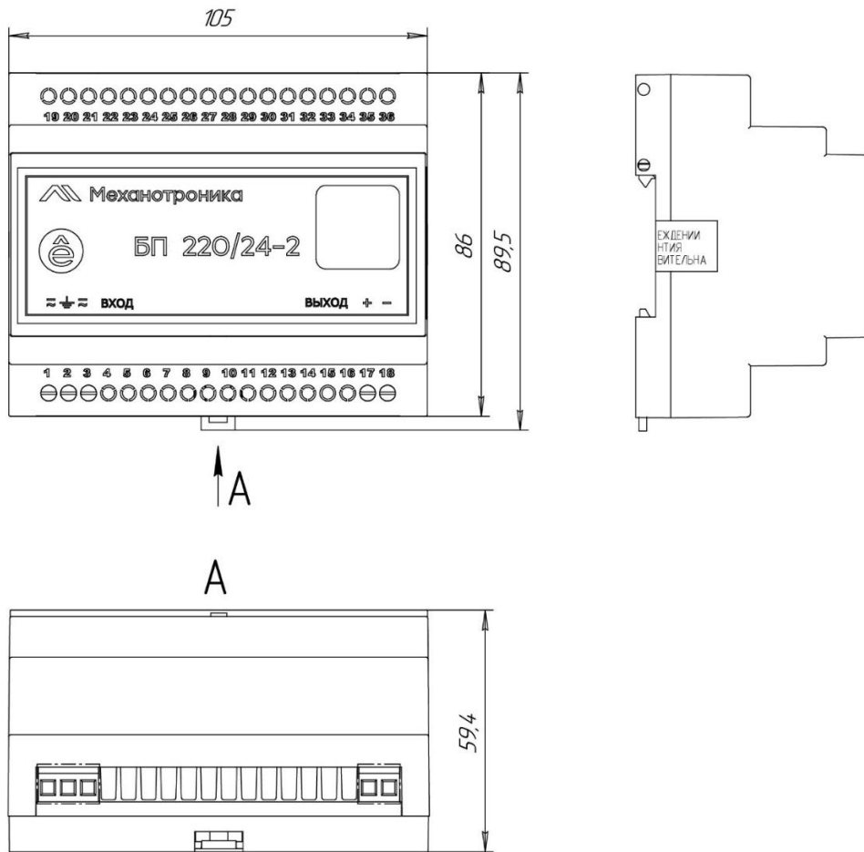
Рисунок 1 – Габаритные размеры
