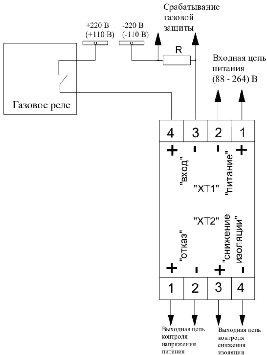
Рисунок 3 – Пример схемы подключения РКИ
