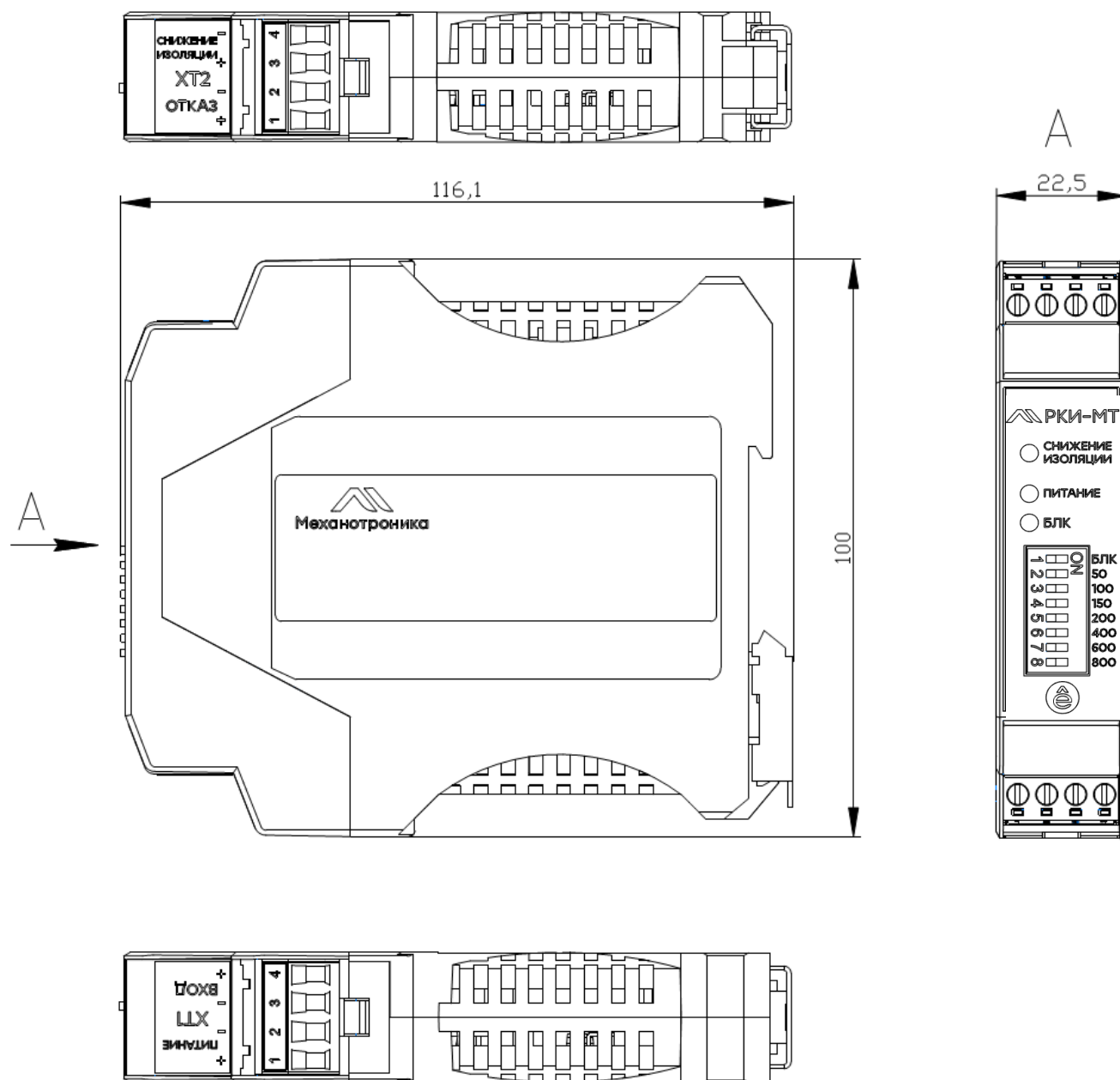
Рисунок 1 – Габаритные размеры и внешний вид РКИ
