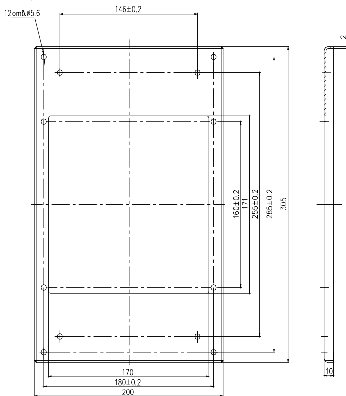
Рисунок 1 - Габаритные, присоединительные и установочные размеры панели
