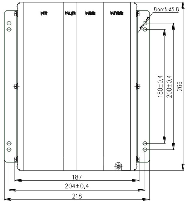
Варианты установки угольников к блоку
