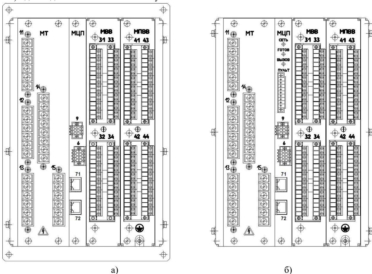
Рисунок 2 – Расположение съемных модулей в исполнениях блока
