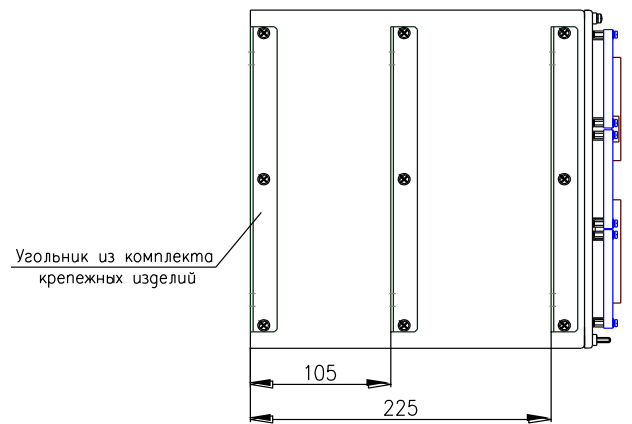
Разметка для крепления блока за основание
