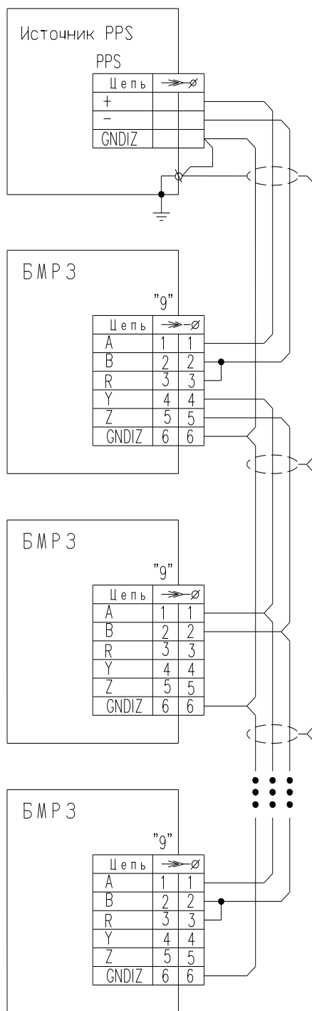
Рисунок Б.3 - Схема электрическая подключения цепей PPS (вариант 1)
