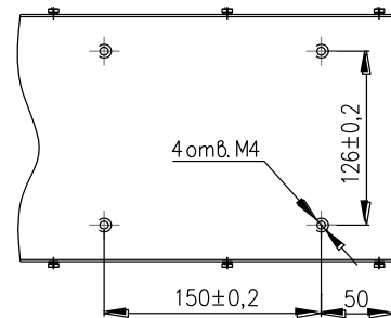
Разметка для крепления блока за основание
