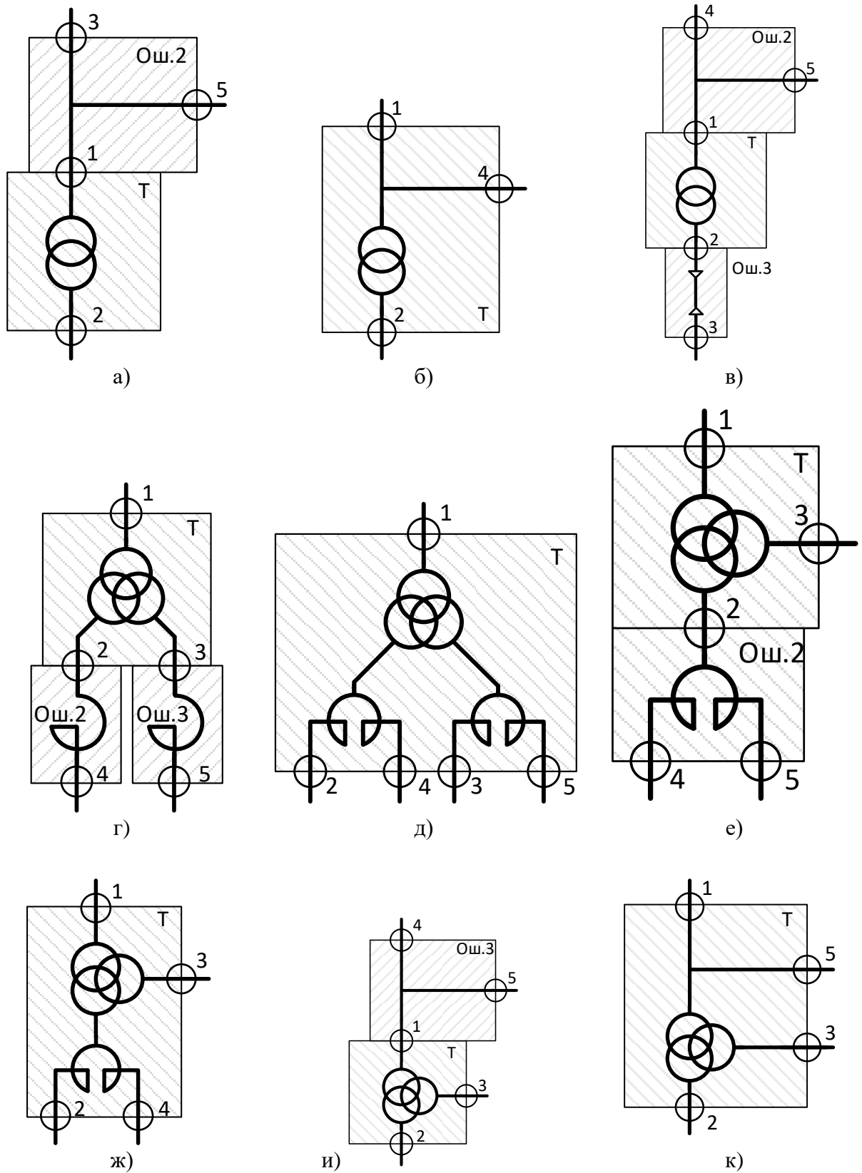
Рисунок 1 (лист 1 из 2) - Примеры распределения зон защиты
