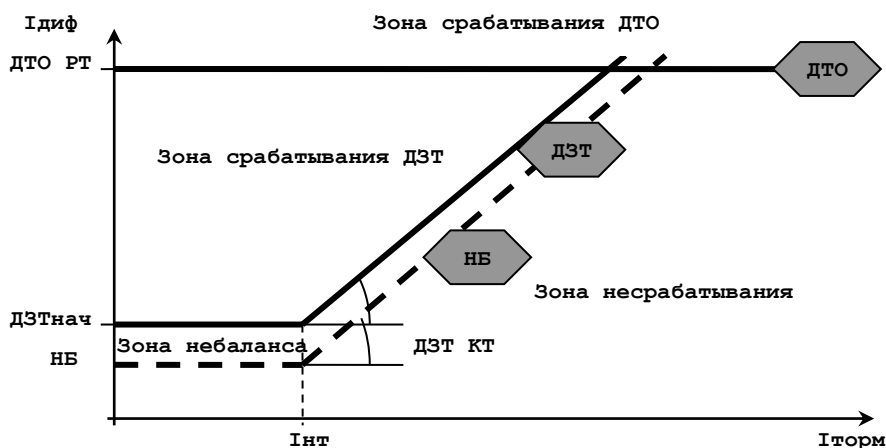
Рисунок 8 - Характеристика срабатывания дифференциальных защит ошиновки
