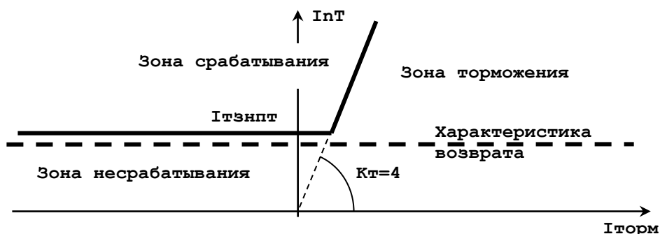
Рисунок 9 - Характеристика срабатывания и возврата ТЗНПТ
