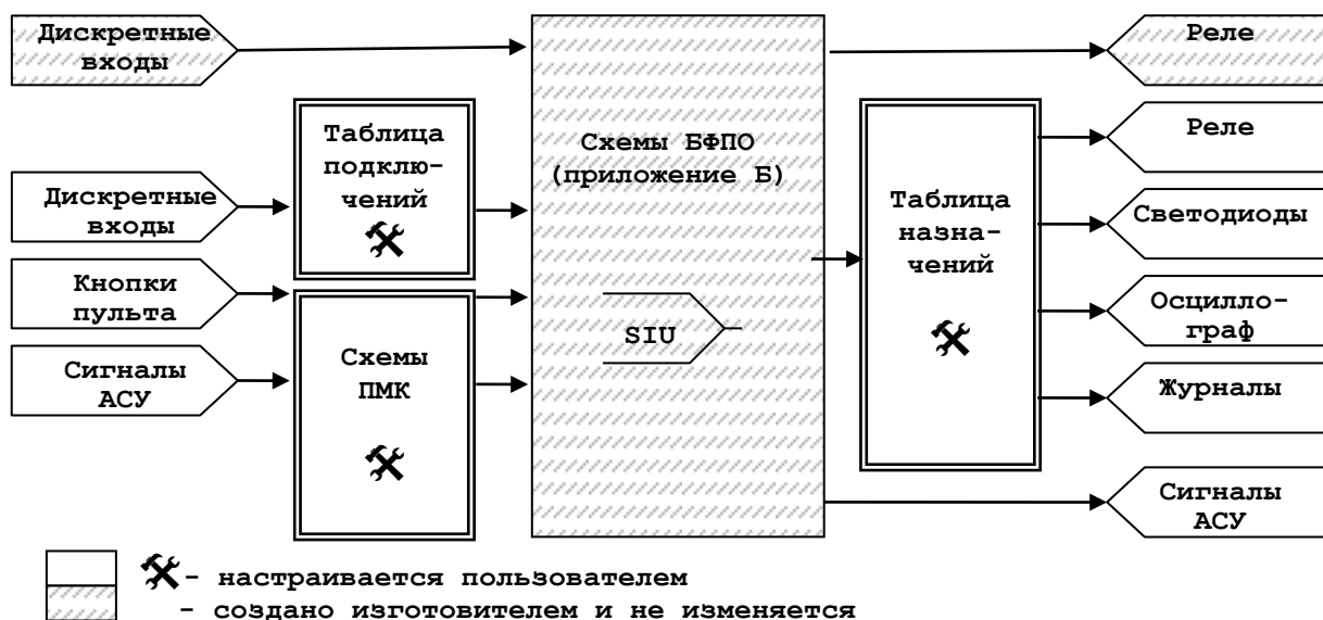
Рисунок 3 - Схема настройки блока
