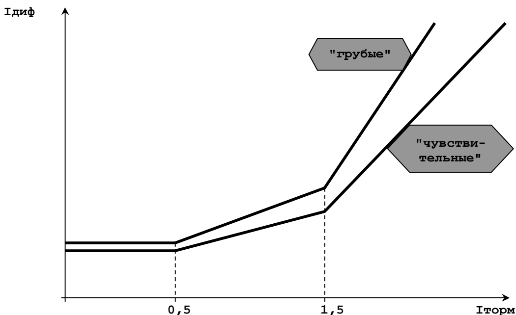
Рисунок 7 - Характеристики срабатывания "грубой" и "чувствительной" ДЗТ
