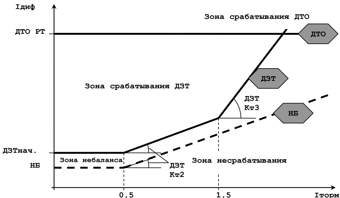
Рисунок 6 - Характеристика срабатывания дифференциальных защит Т (АТ)
